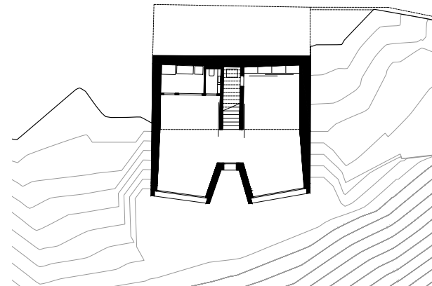
Rez inférieur
